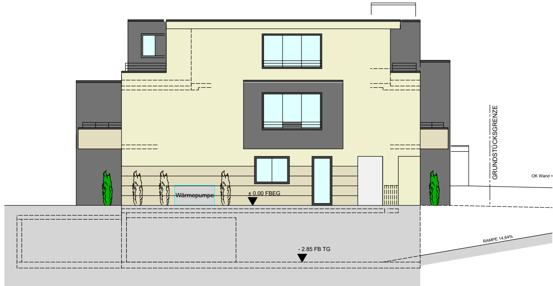
ANSICHT NORD-WEST
